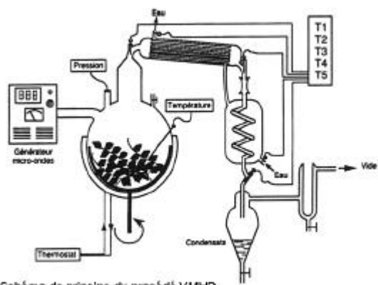
Schéma de principe du procédé VMHD
